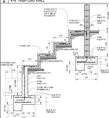
1 SECTION A-A
